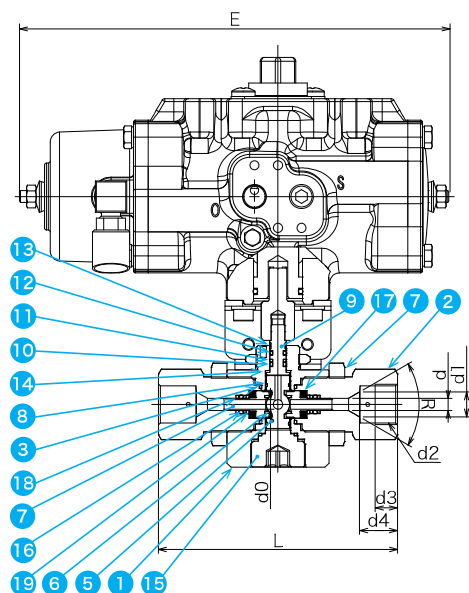
■寸法表
