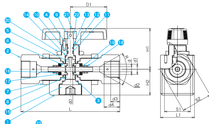
■寸法表
