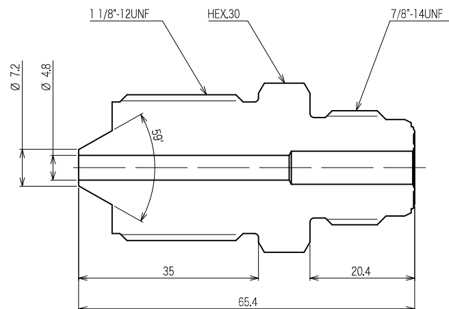
型 式 CJ-HCVC8R-9CS60
