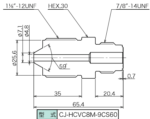
C&T(1 1/8-12UNF)-HCVC変換継手
