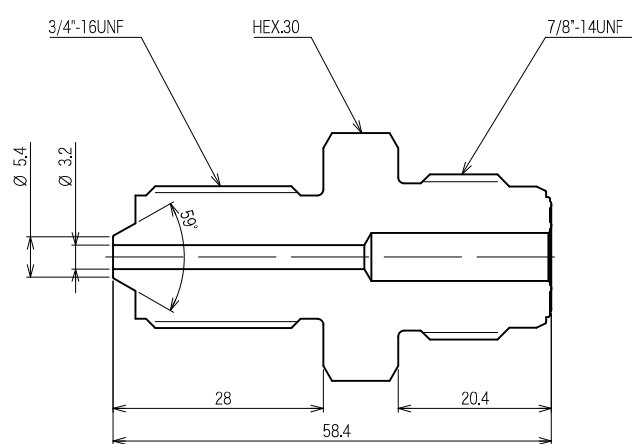
型 式 CJ-HCVC8R-6CS60
